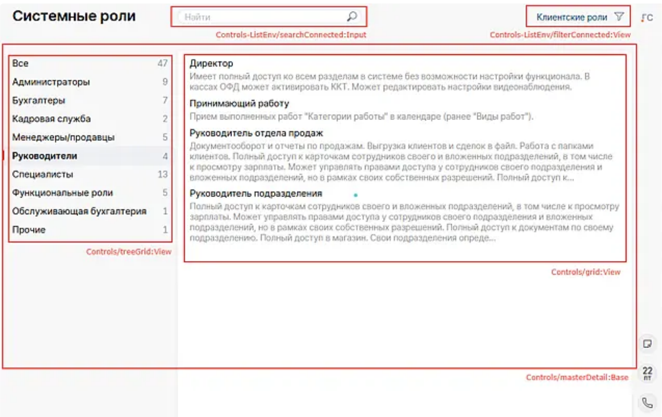
Рисунок 1. Декомпозиция интерфейса «Рееестр системных ролей»
