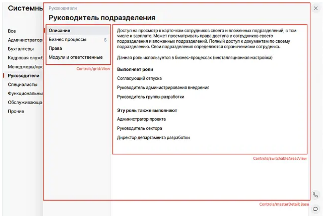
Рисунок 2. Декомпозиция интерфейса «Карточка системной роли»
